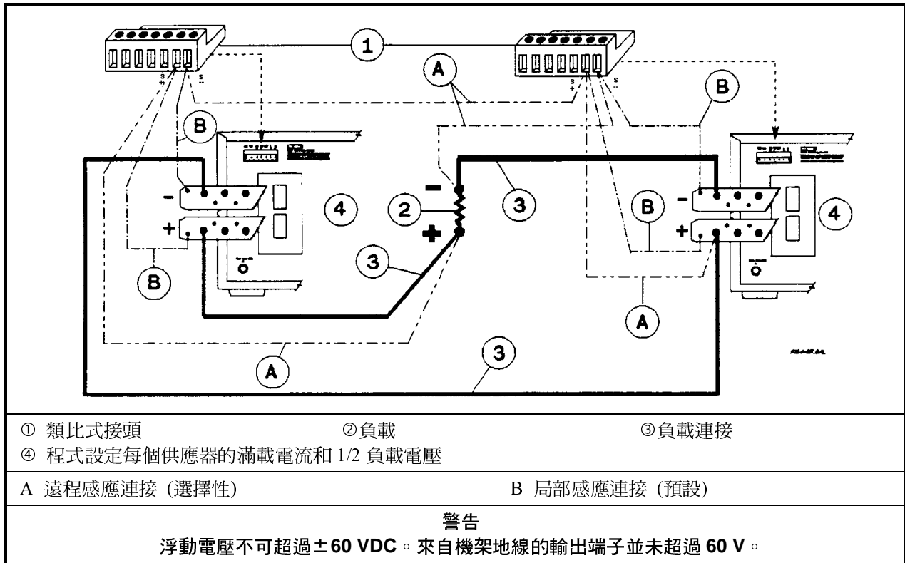
圖 6e：型號 668xA 的串聯 (遠程感應選用配備)
