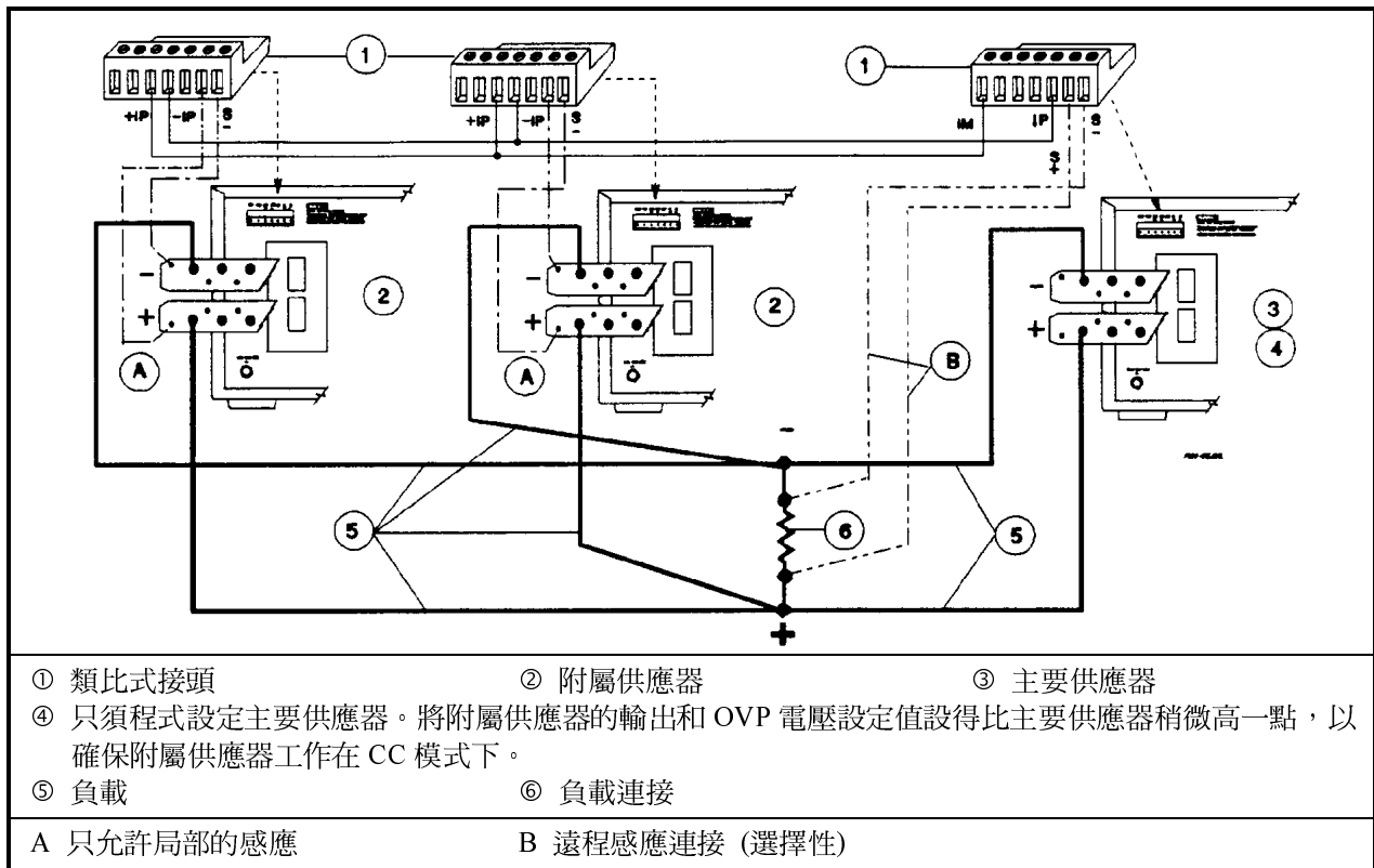
圖 6d : 型號 668xA 自動並聯 (遠程感應選用配備)
