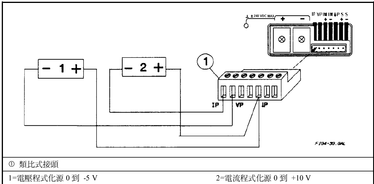
圖 4f：654xA、655xA、664xA 和 666xA 系列類比程式化連接
