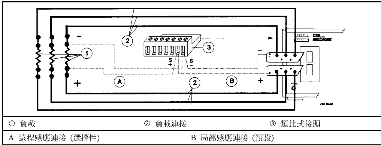
圖 6c : 型號 668xA 多個負載連接 (遠程感應選用配備)
