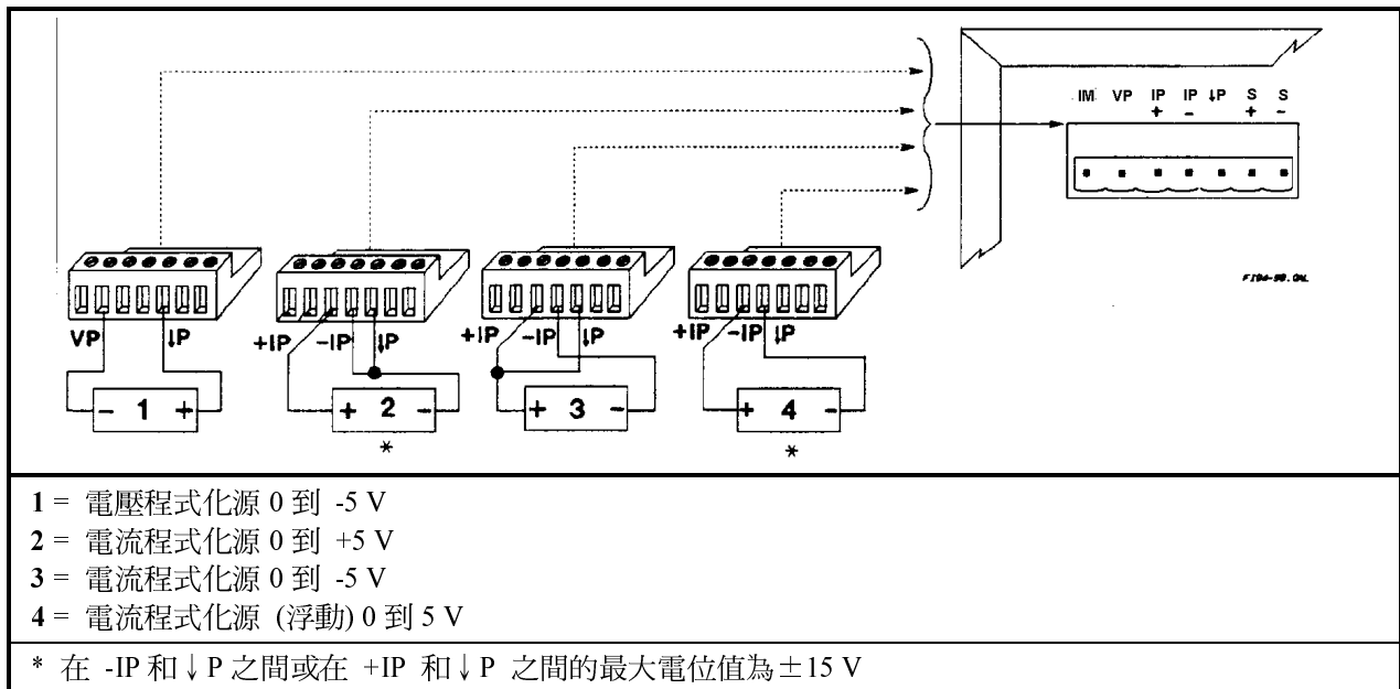
圖 6f：型號 668xA 類比程式化連接
